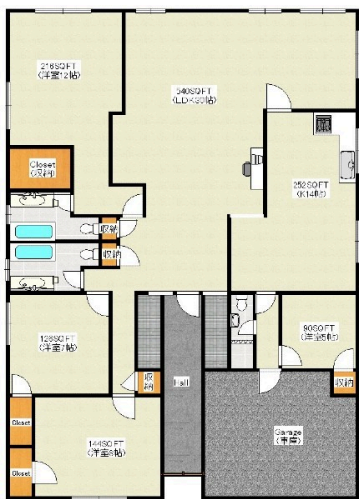
【間取り図】
