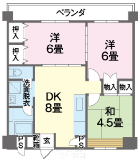
【間取り図】
