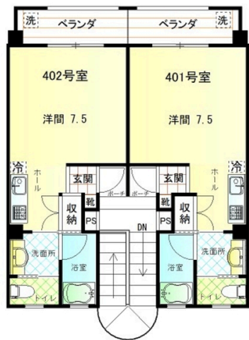
【間取り図】
