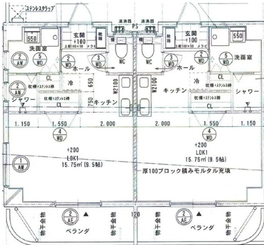
【間取り図】
