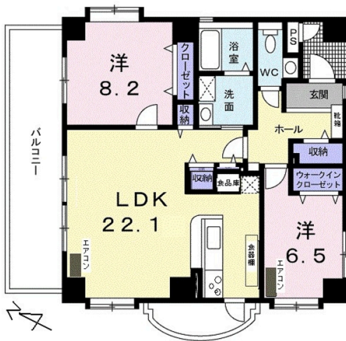
【間取り図】
