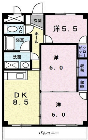
【間取り図】
