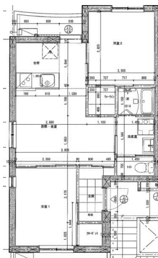
【間取り図】
