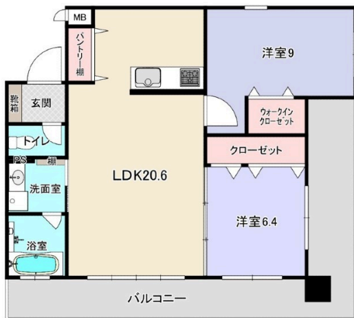
【間取り図】
