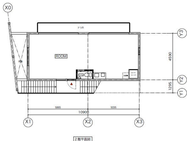
【間取り図】
