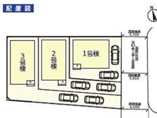
配置図
