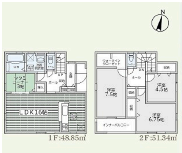
【間取り図】
