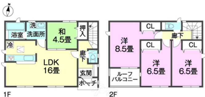
【間取り図】
