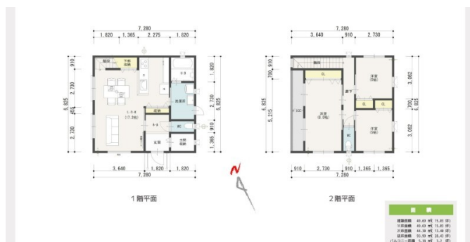
【間取り図】
