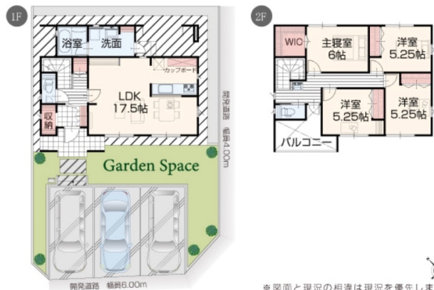
18号棟間取図
