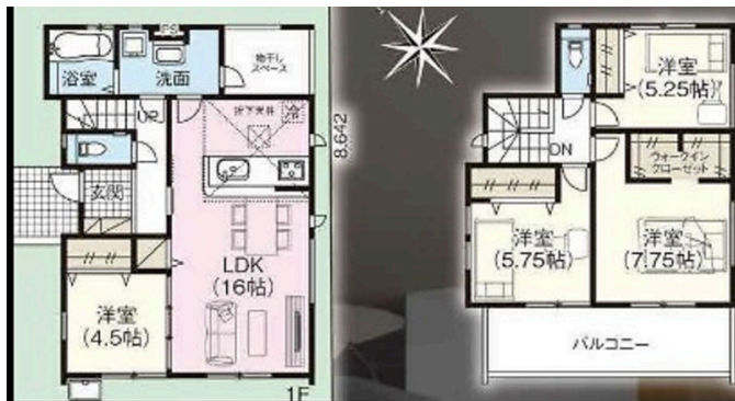
【間取り図】
