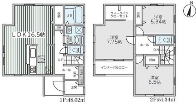
【間取り図】
