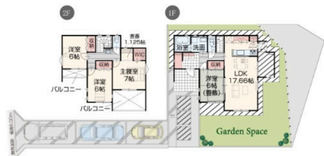
20号棟間取図
