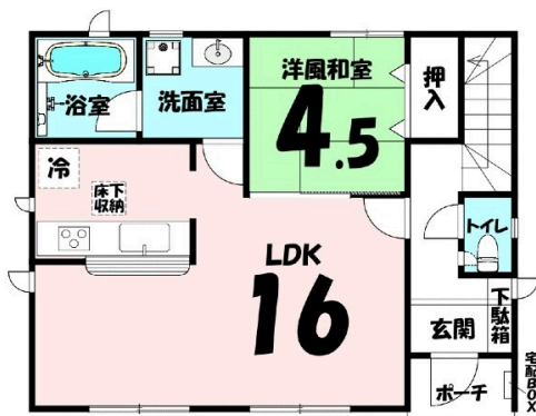
1階平面図
