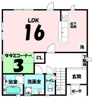
1階平面図
