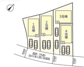
配置図
