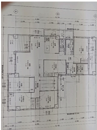
【間取り図】
