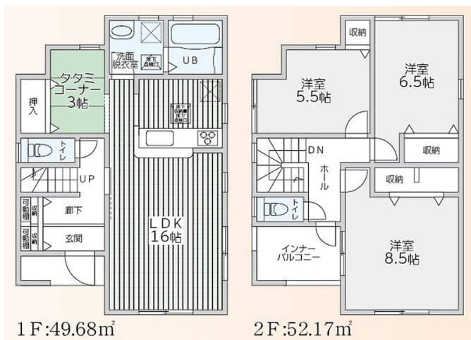
【間取り図】
