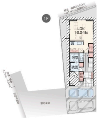
2号棟間取図
