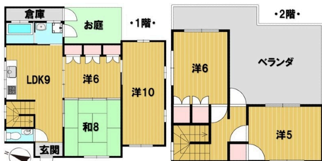
【間取り図】
