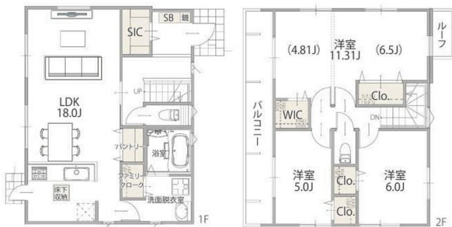
【間取り図】
