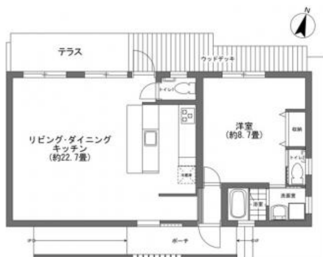
【間取り図】
