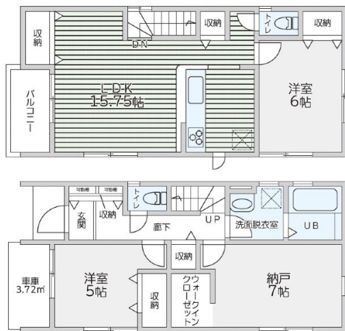
【間取り図】
