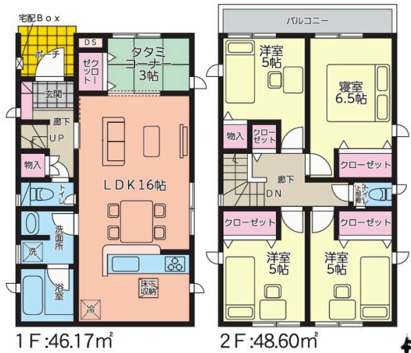
【間取り図】
