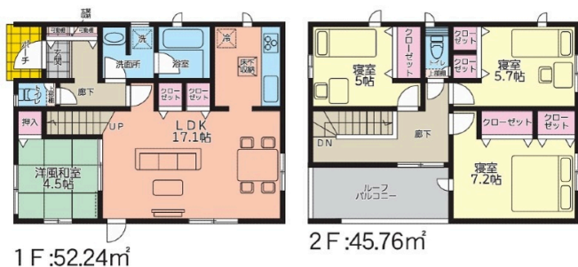
【間取り図】
