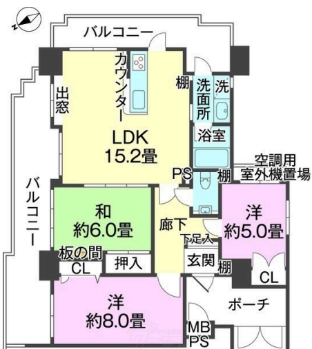
【間取り図】
