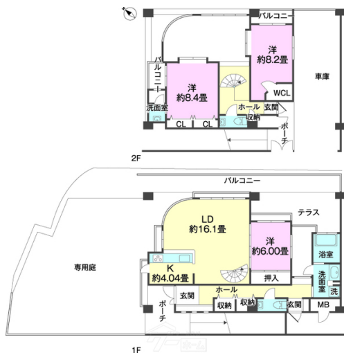
【間取り図】
