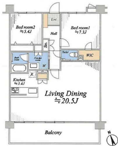
【間取り図】
