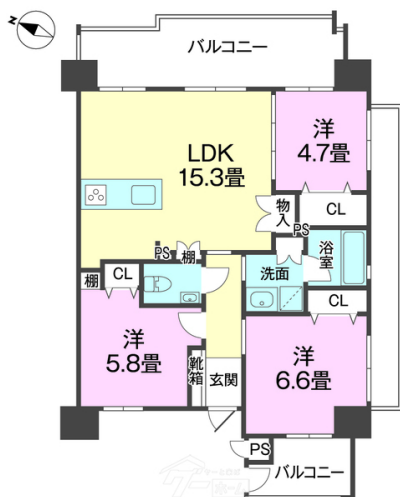
【間取り図】
