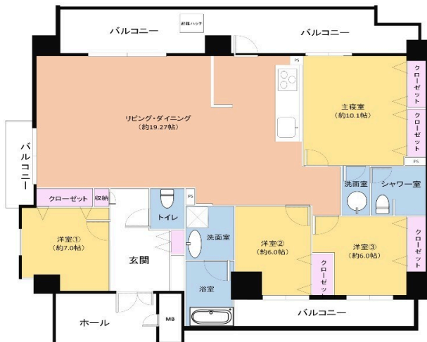
【間取り図】
