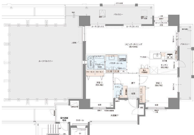
【間取り図】
